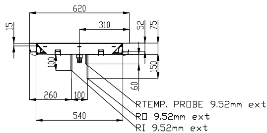
Zij aanzicht
