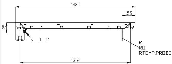
Zij aanzicht
