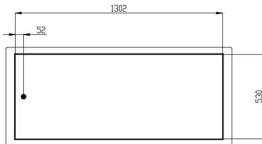
Boven aanzicht
